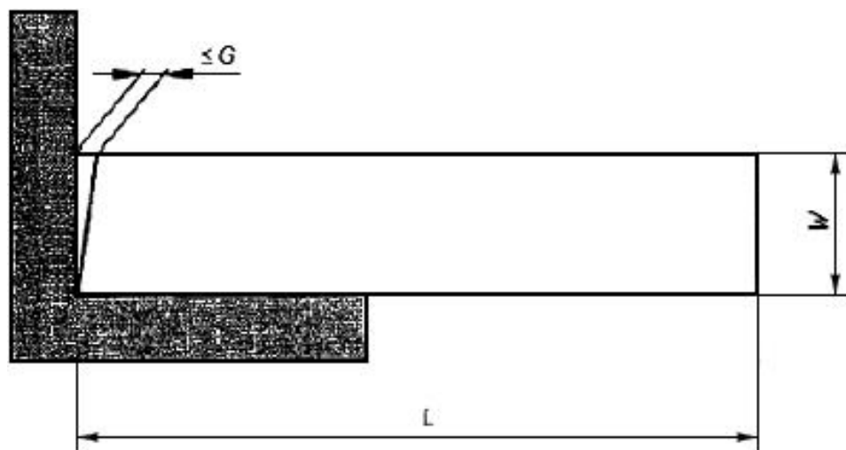
Рисунок А.4 - Определение прямоугольности G
