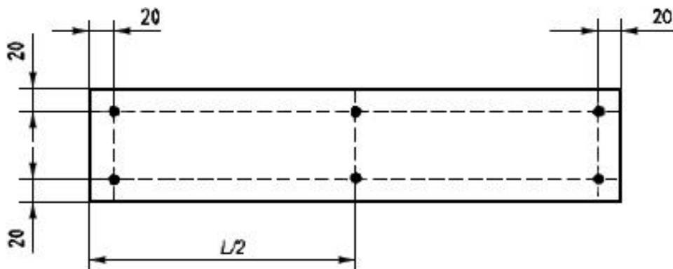
Рисунок А.3 - Точки измерения для определения толщины ( T , размеры в мм)
