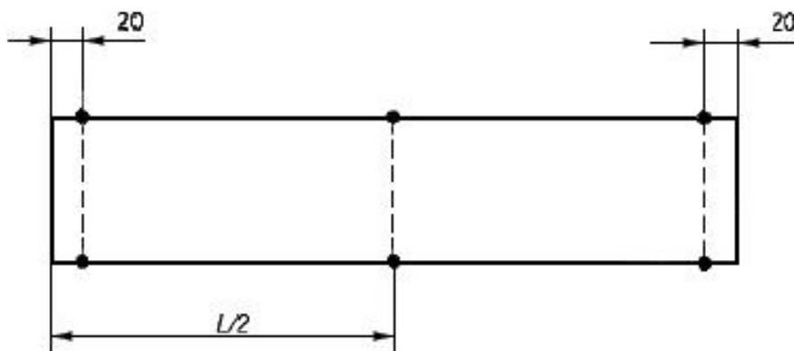
Рисунок А.2 - Точки измерения для определения ширины ( W , размеры в мм)
