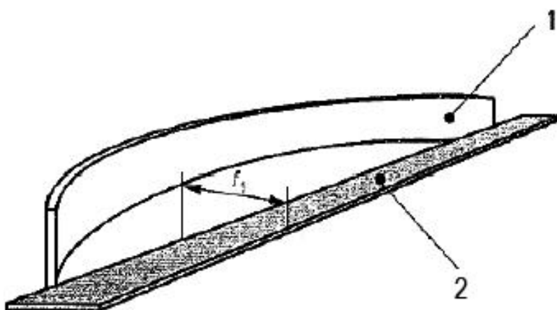
Рисунок А.7 - Определение покоробленности по длине f_1
