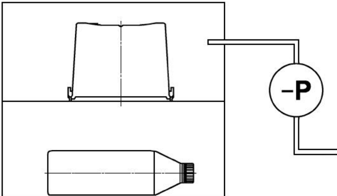
Рисунок 1 - Контроль герметичности тары в вакуумной камере
